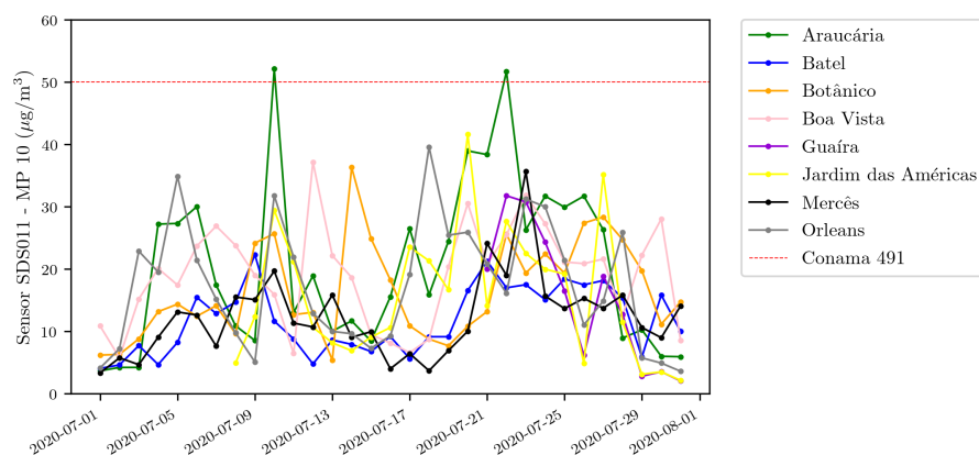
Figura 3.2: Médias diárias de MP_{10} dos pontos de amostragem para julho de 2020.
