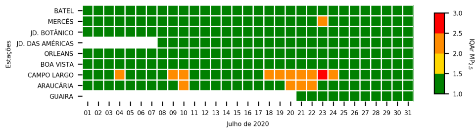
Figura 3.10: IQAr baseado na concentração diária de MP_{2.5} em todos os pontos amostrais
