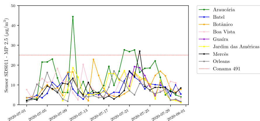
Figura 3.1: Médias diárias de MP_{2,5} dos pontos de amostragem para julho de 2020.
