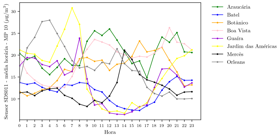
Figura 3.4: Perfis diários de MP 10 dos pontos de amostragem para julho de 2020
