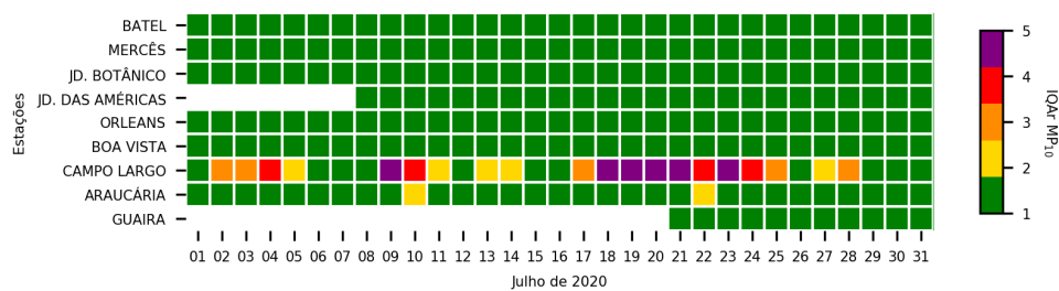
Figura 3.11: IQAr baseado na concentração diária de MP_{10} em todos os pontos amostrais
