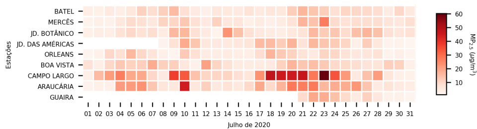
Figura 3.8: Concentração média diária de MP_{2.5} em todos os pontos amostrais
