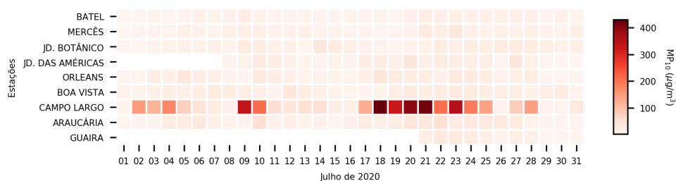
Figura 3.9: Concentração média diária de MP_{10} em todos os pontos amostrais
