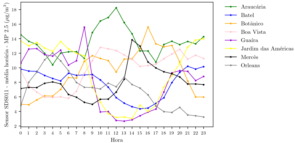
Figura 3.3: Perfis diários de MP 2,5 dos pontos de amostragem para julho de 2020
