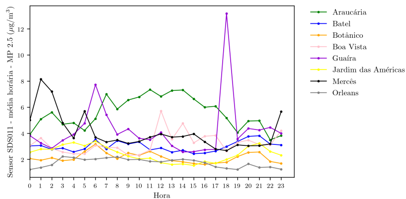
Figura 3.3: Perfis diários de MP_{2,5} dos pontos de amostragem para dezembro de 2020
