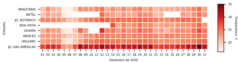
Figura 3.8: Temperatura média diária nos pontos amostrais
