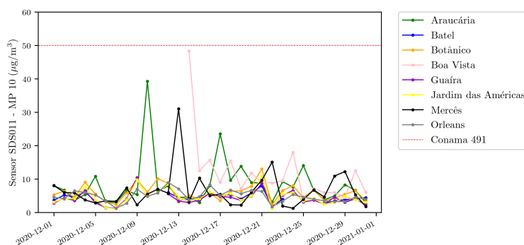
Figura 3.2: Médias diárias de MP 10 dos pontos de amostragem para dezembro de 2020.
