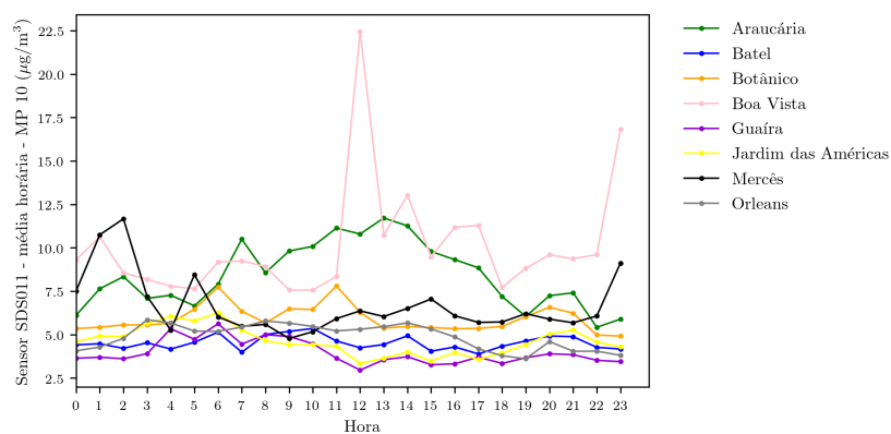
Figura 3.4: Perfis diários de MP_{10} dos pontos de amostragem para dezembro de 2020
