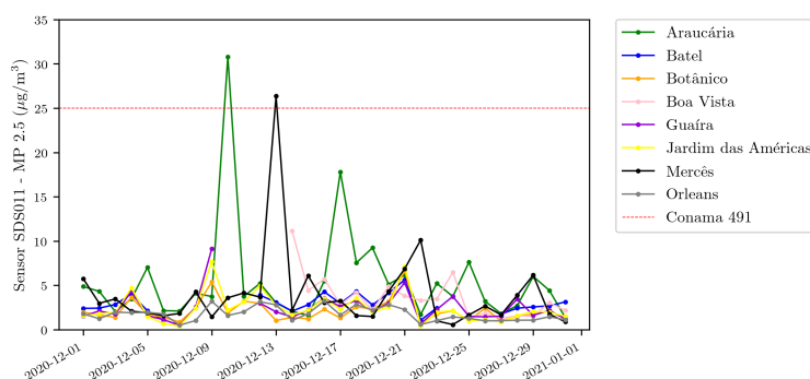
Figura 3.1: Médias diárias de MP 2,5 dos pontos de amostragem para dezembro de 2020.
