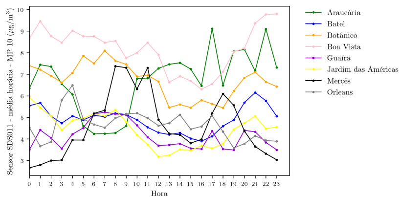
Figura 3.4: Perfis diários de MP 10 dos pontos de amostragem para janeiro de 2021
