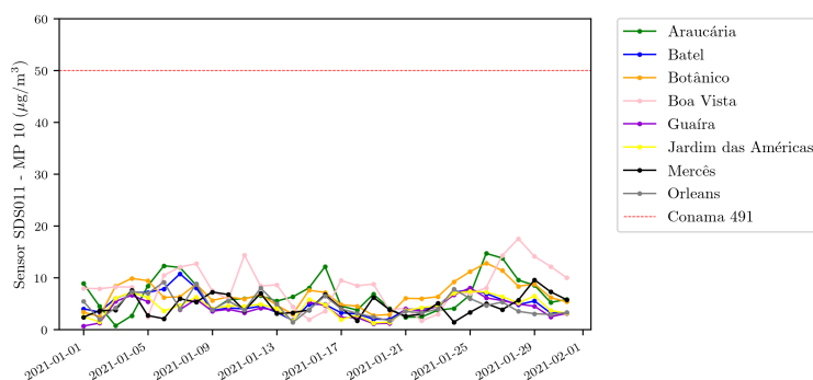
Figura 3.2: Médias diárias de MP_{10} dos pontos de amostragem para janeiro de 2021.
