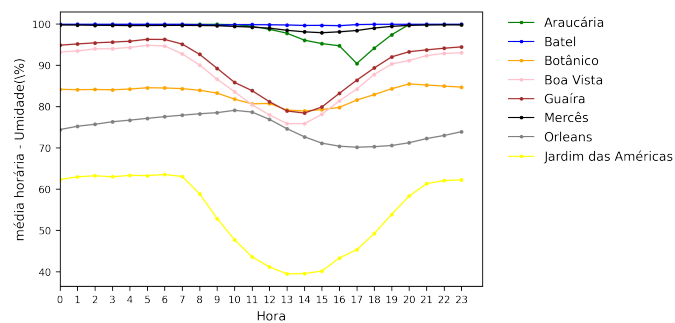
Figura 3.7: Perfil diário de umidade horária média nos pontos amostrais
