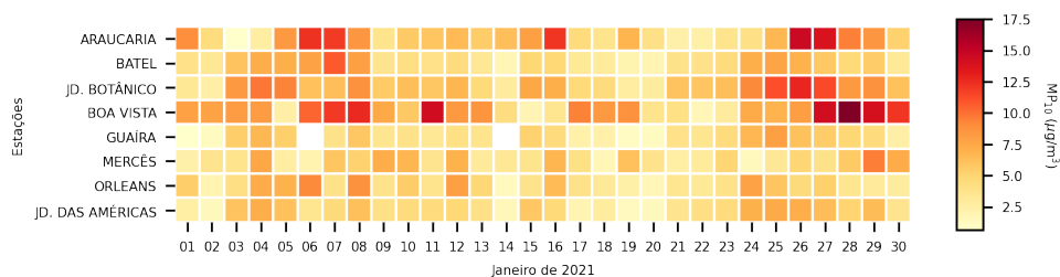
Figura 3.12: Concentração média diária de PM_{10} em todos os pontos amostrais
