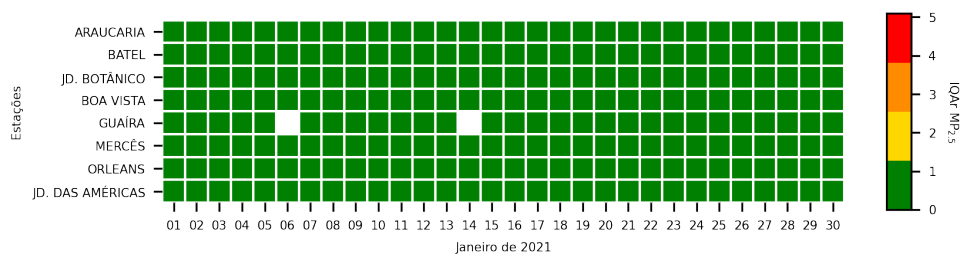
Figura 3.13: IQAr baseado na concentração diária de PM_{2.5} em todos os pontos amostrais
