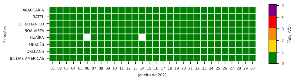
Figura 3.14: IQAr baseado na concentração diária de PM_{10} em todos os pontos amostrais
