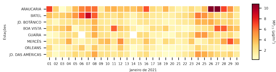
Figura 3.11: Concentração média diária de PM_{2.5} em todos os pontos amostrais
