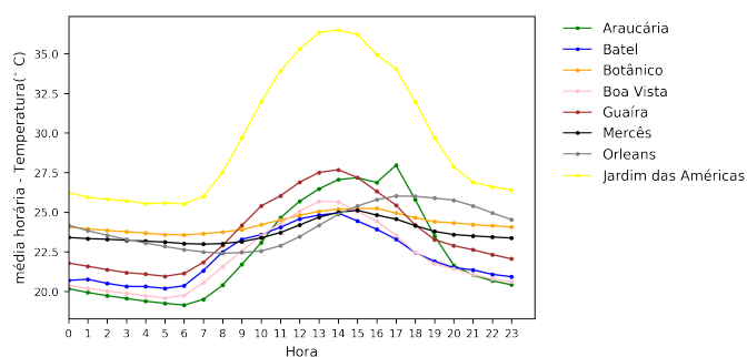
Figura 3.6: Perfil diário de temperatura horária média nos pontos amostrais
