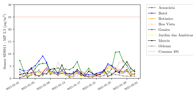
Figura 3.1: Médias diárias de MP_{2,5} dos pontos de amostragem para janeiro de 2021.
