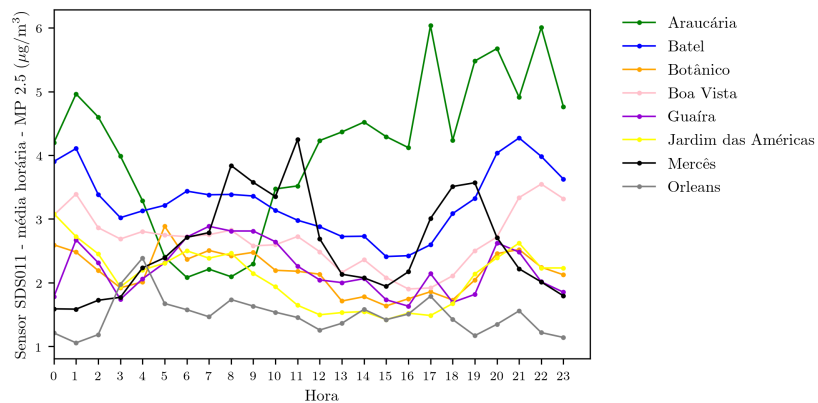
Figura 3.3: Perfis diários de MP 2,5 dos pontos de amostragem para janeiro de 2021
