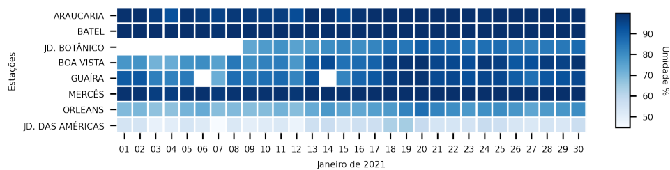
Figura 3.9: Umidade média diária nos pontos amostrais
