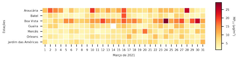
Figura 3.11: Concentração média diária de MP_{10} em todos os pontos amostrais
