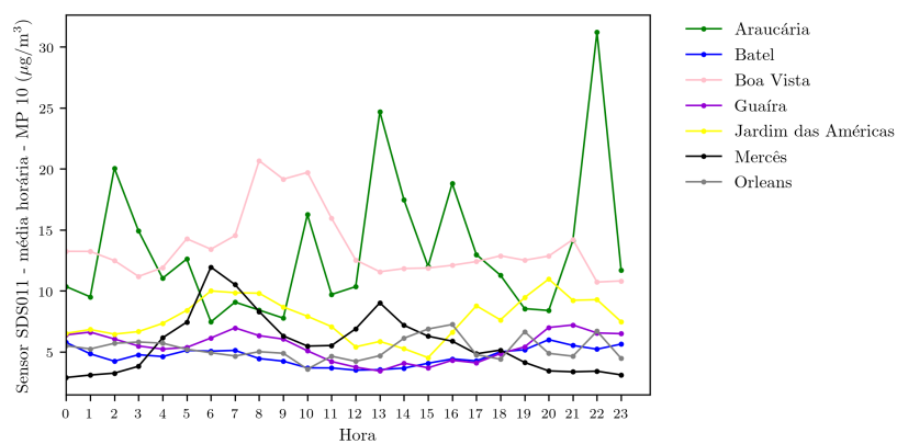
Figura 3.4: Perfis diários de MP 10 dos pontos de amostragem para março de 2021
