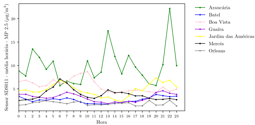
Figura 3.3: Perfis diários de MP 2,5 dos pontos de amostragem para março de 2021
