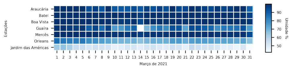
Figura 3.8: Umidade média diária nos pontos amostrais
