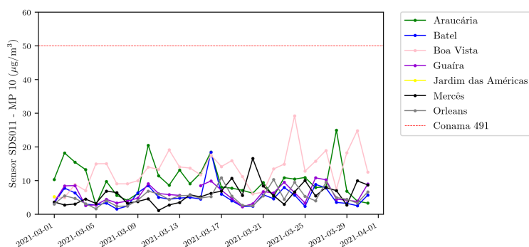
Figura 3.2: Médias diárias de MP 10 dos pontos de amostragem para março de 2021.
