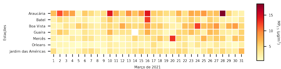
Figura 3.10: Concentração média diária de MP_{2.5} em todos os pontos amostrais
