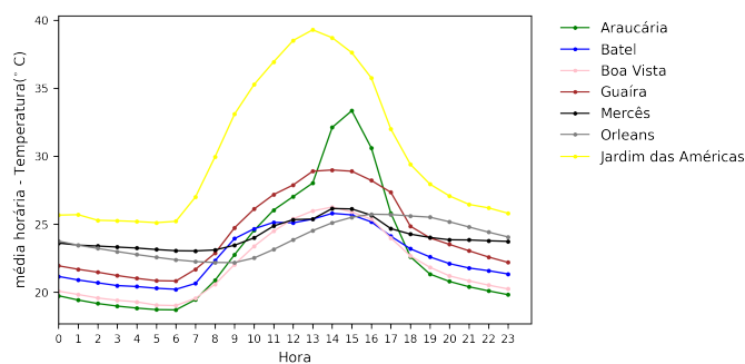
Figura 3.5: Perfil diário de temperatura horária média nos pontos amostrais
