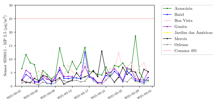
Figura 3.1: Médias diárias de MP 2,5 dos pontos de amostragem para março de 2021.
