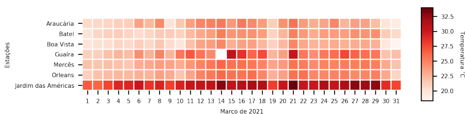
Figura 3.7: Temperatura média diária nos pontos amostrais
