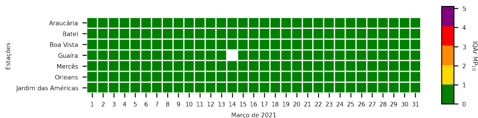
Figura 3.13: IQAr baseado na concentração diária de MP_{10} em todos os pontos amostrais
