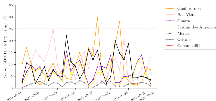
Figura 3.1: Médias diárias de MP_{2,5} dos pontos de amostragem para setembro de 2021.
