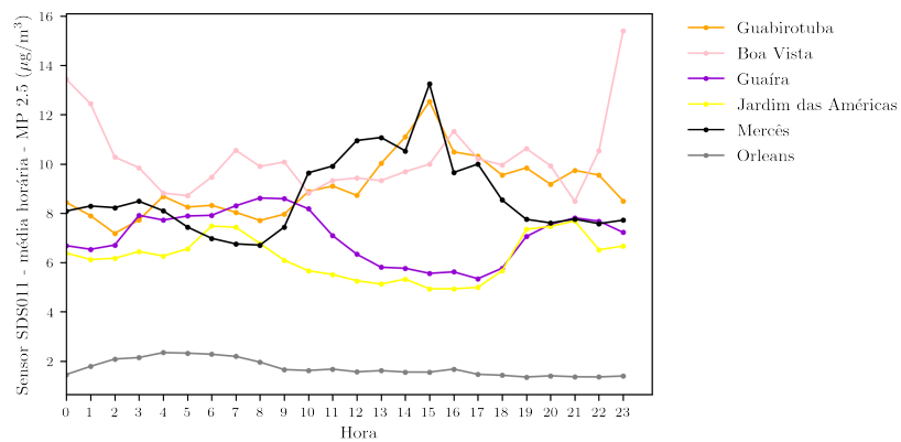
Figura 3.3: Perfis diários de MP_{2,5} dos pontos de amostragem para setembro de 2021
