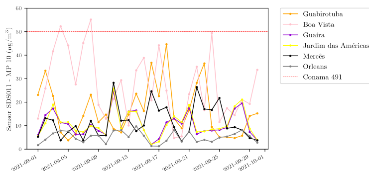
Figura 3.2: Médias diárias de MP_{10} dos pontos de amostragem para setembro de 2021.
